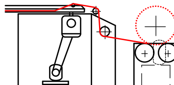
Выход машины для накатки малого диаметра
