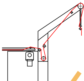
Складывающее устройство № 941 100 902
