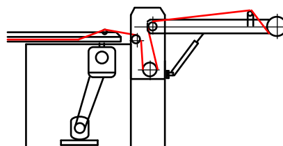
Устройство для накатки большого диаметра № 941 100 901
